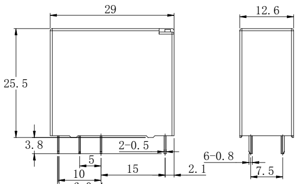
外形尺寸图
