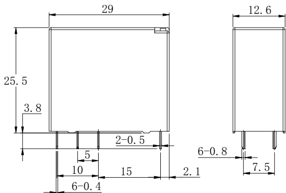
外形尺寸图
