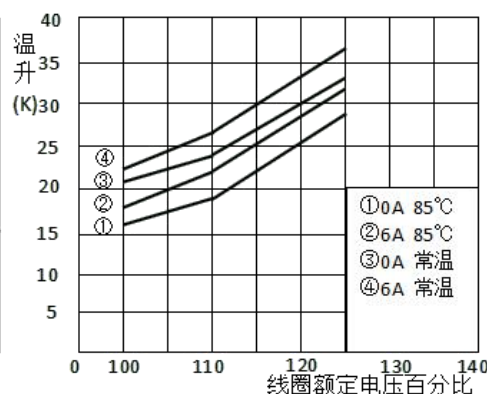
线圈温升
