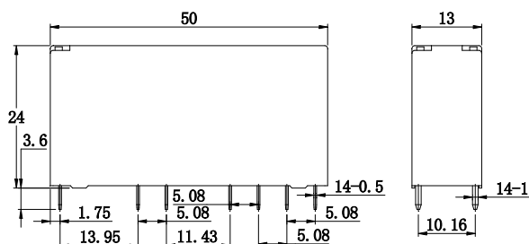
外形尺寸图
