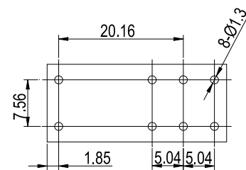
(底视图)
