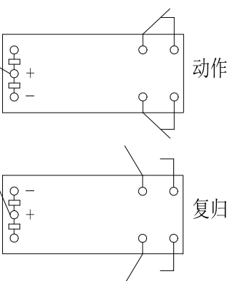
接线图
