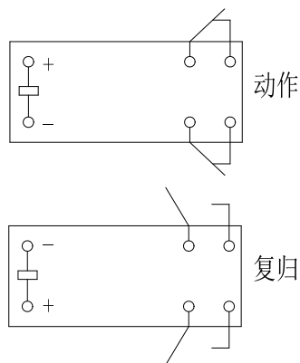
接线图
