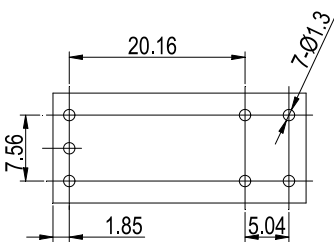
(底视图)
