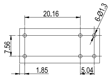
(底视图)
