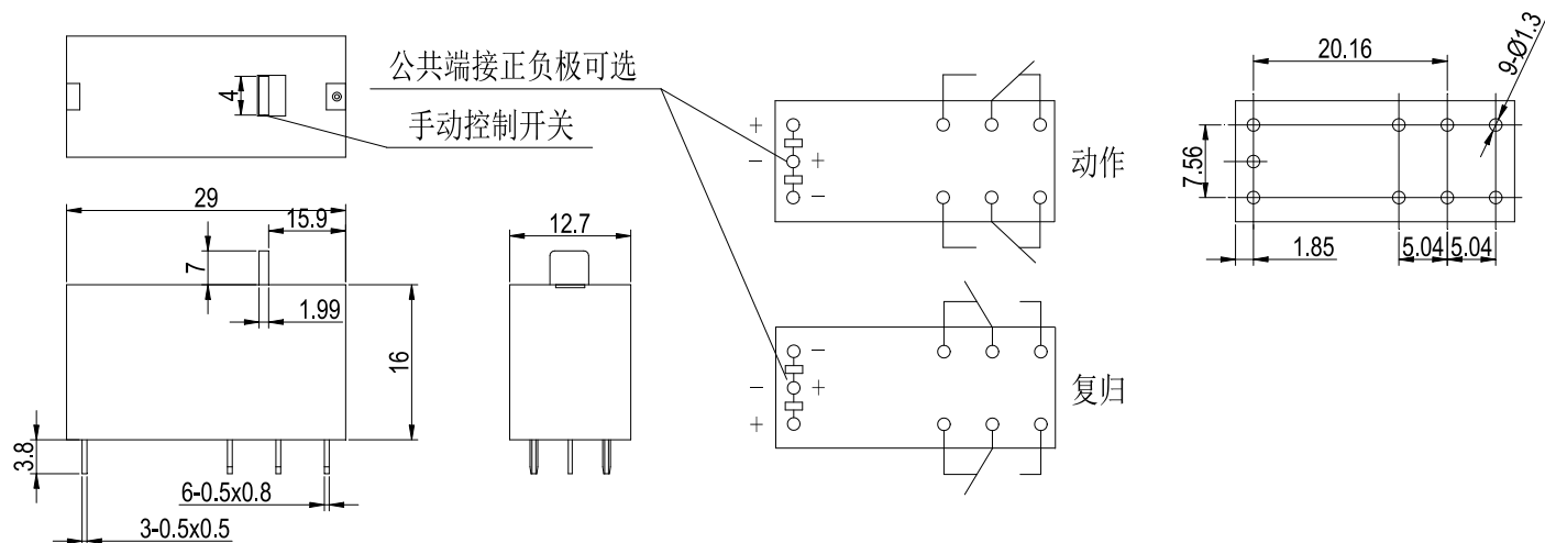
2C(双线圈)
