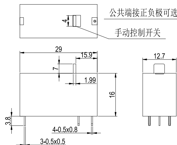
2C(单线圈)
