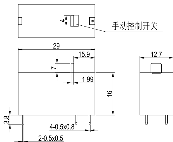
2A/2B(双线圈)
