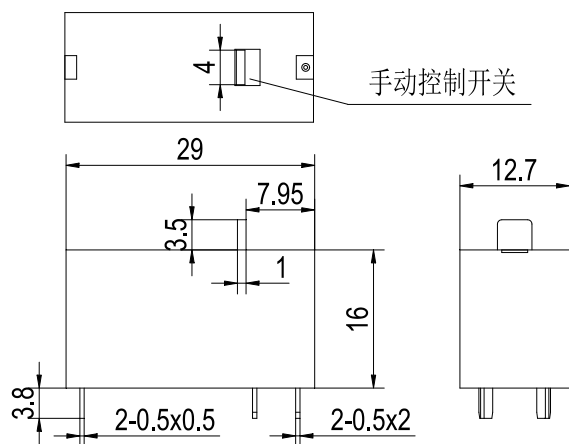
1A1/1B1(双线圈)
