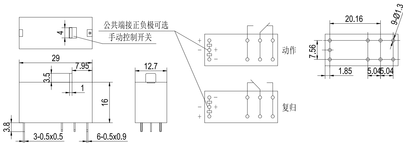
1C2(双线圈)
