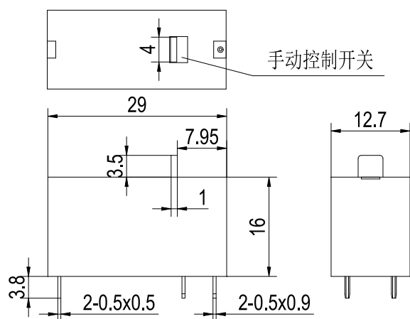
1A5/1B5(双线圈)
