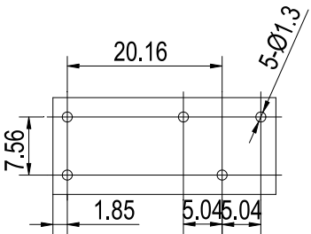
(底视图)
