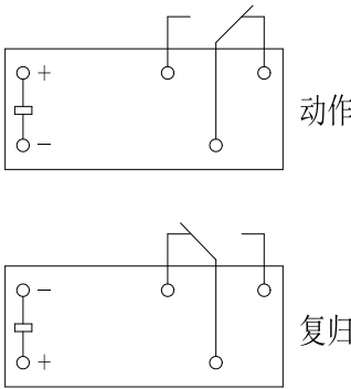
接线图
