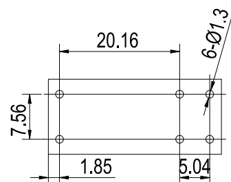
安装尺寸图
