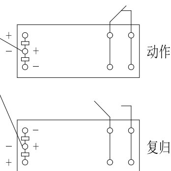
接线图
