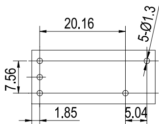
(底视图)
