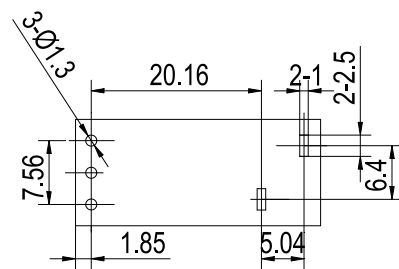
安装尺寸图
