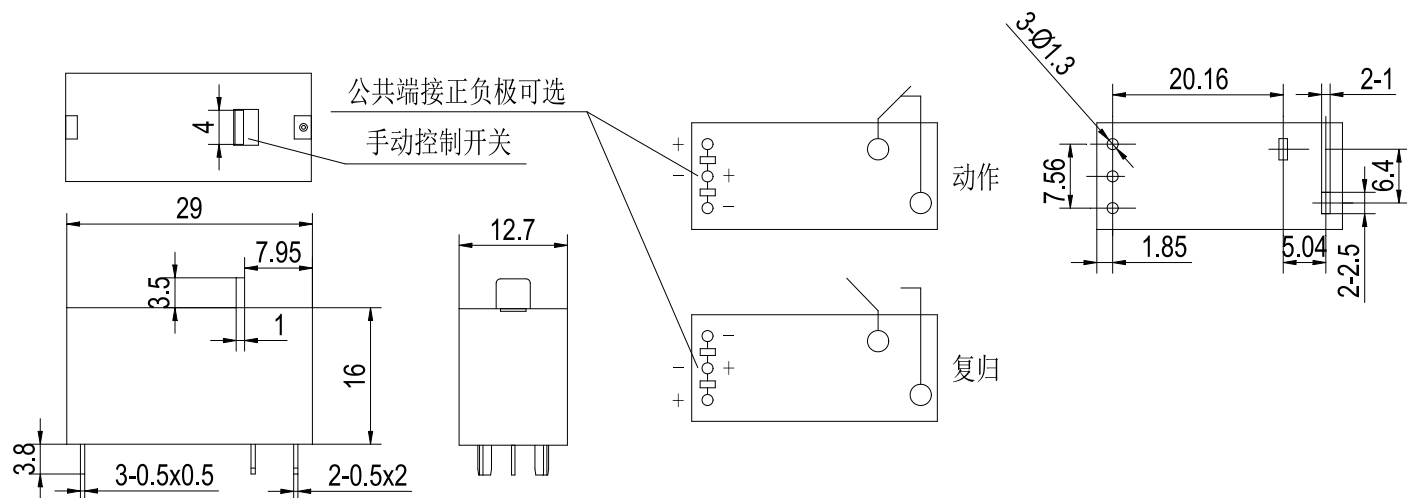
1C2(单线圈)
