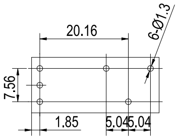
(底视图)
