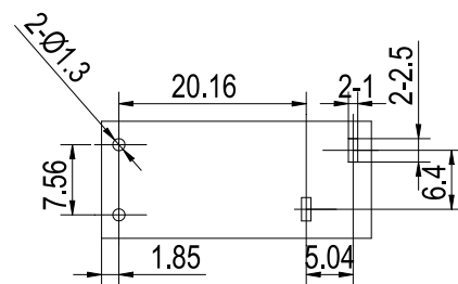
安装尺寸图
