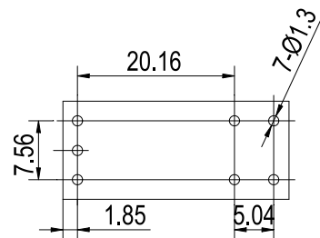
安装尺寸图
