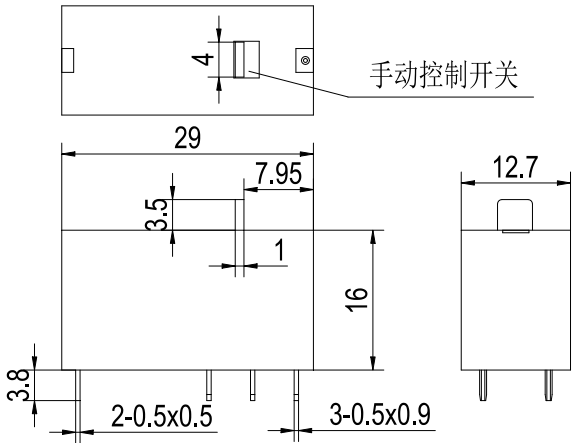
1C5(双线圈)
