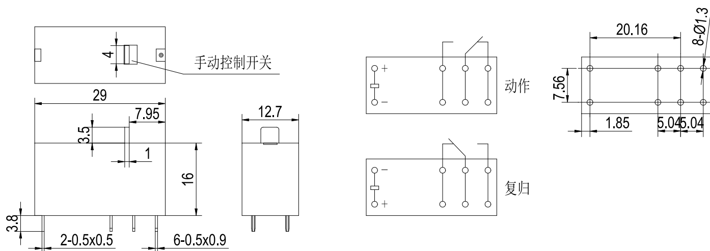
1C2(双线圈)
