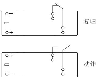
接线图 (底视图)
