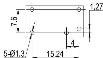
安装尺寸图
