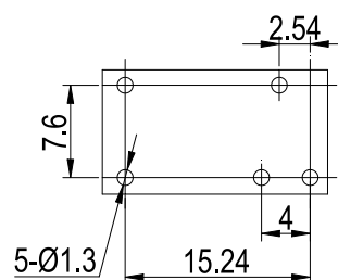
安装尺寸图
