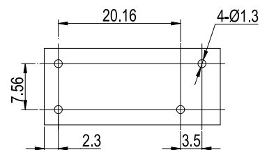
安装尺寸图
