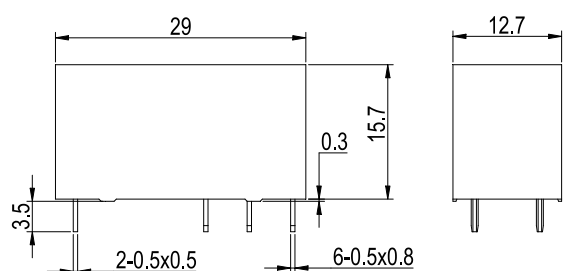
外形尺寸图
