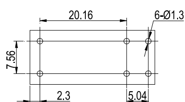
安装尺寸图
