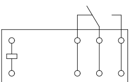
接线图
