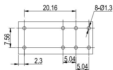
安装尺寸图
