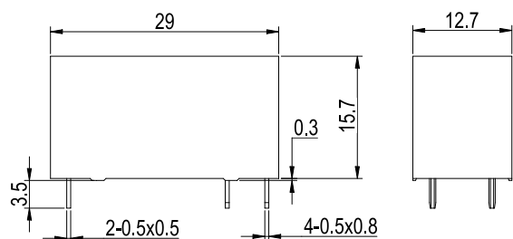
外形尺寸图
