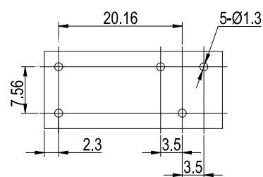
安装尺寸图
