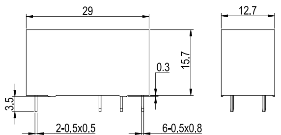
外形尺寸图
