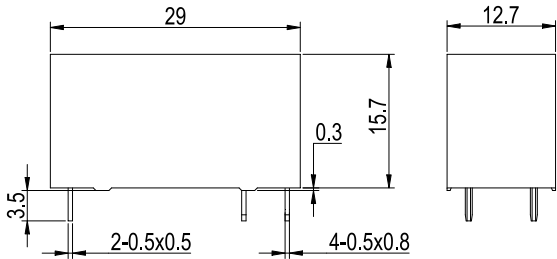
外形尺寸图
