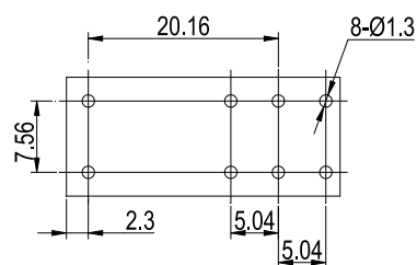
安装尺寸图
