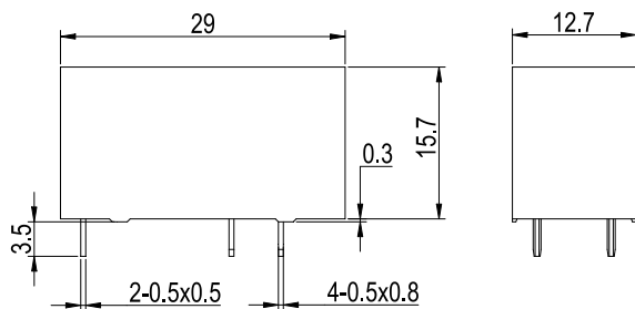
外形尺寸图
