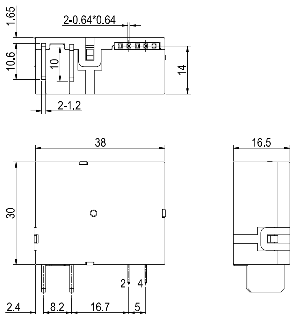
A 型单线圈
