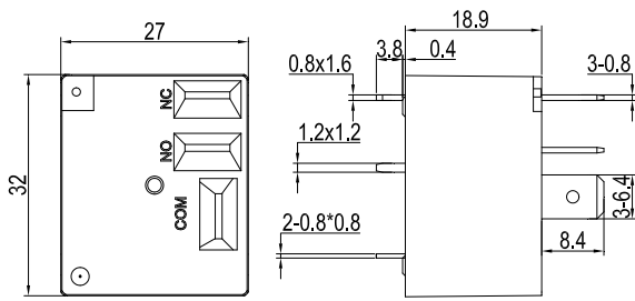
1C 外形尺寸图
