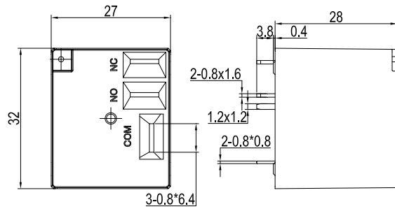
1C(H2) 外形尺寸图
