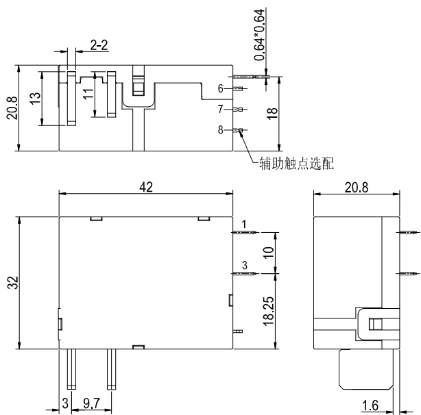
A 型单线圈
