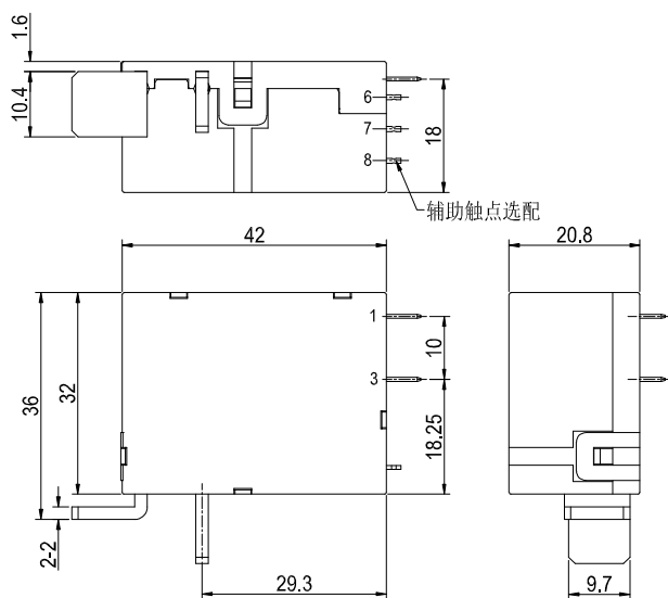
B 型单线圈
