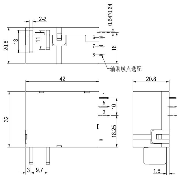
A 型双线圈
