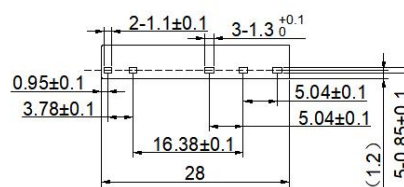
(底视图)
